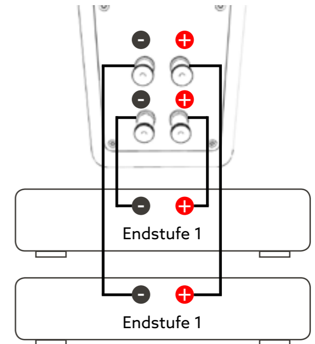
Bi-Amping
