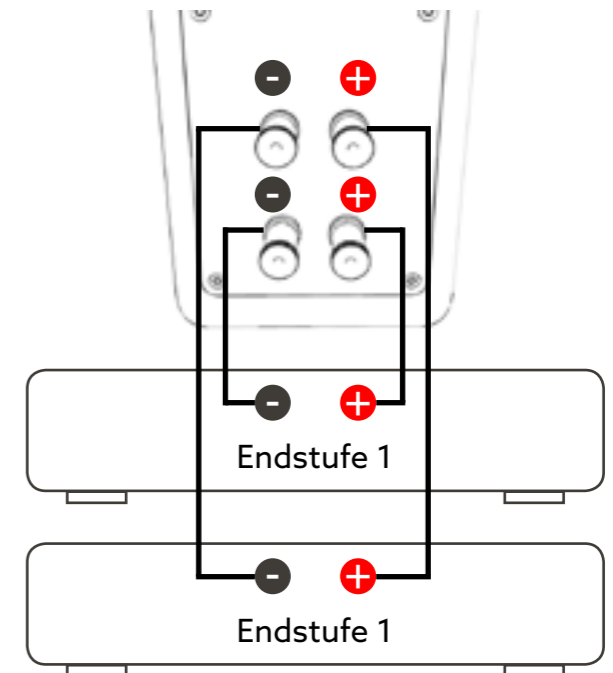
Bi-Amping
